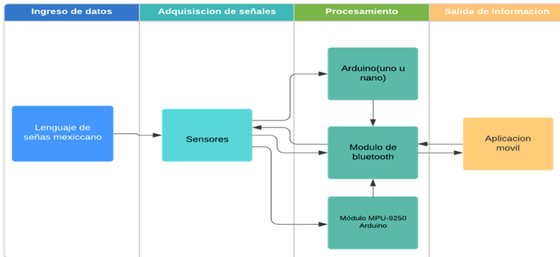
Fig. 12. Diagrama de bloques del funcionamiento del dispositivo wearable para la traducción de lenguaje de señas mexicano.
