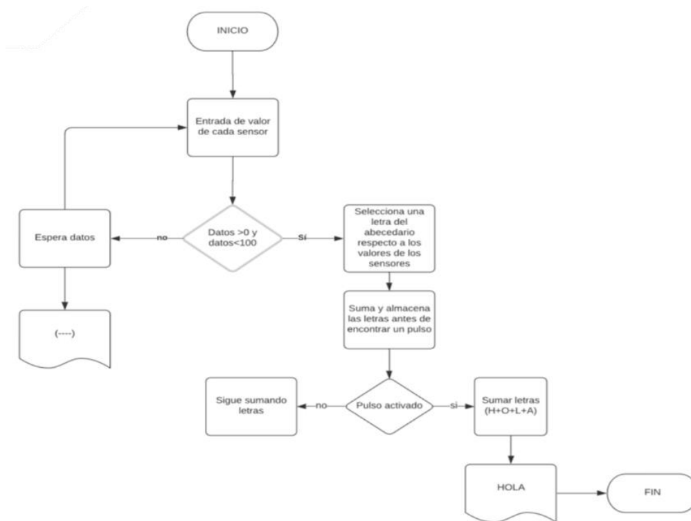
Fig. 11. Diagrama de flujo de la interacción del código al introducir más de una letra del alfabeto.
