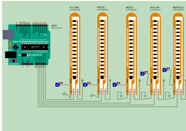
Fig. 8. Simulación en Proteus de los sensores flexibles conectados al Arduino UNO.
