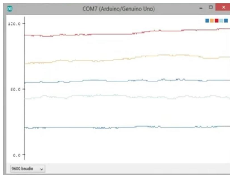
Fig. 9. Impresión de pantalla del puerto serial de 0 a 1000 Ohm.
